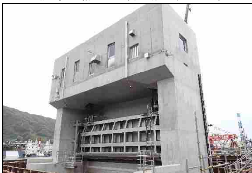
津波から市街地を防護する水門 (和歌山下津港海岸)
