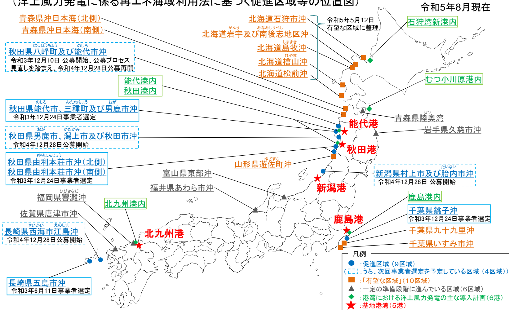
秋田港内洋上風力発電事業
